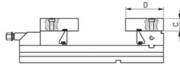
Увеличенной длины Art.136 - закаленные; Art. 136S - мягкие.
