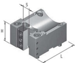
Резцедержатель для наружной обработки Рисунок 3
