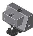
Кулачок с установочным прижимом Art.615
