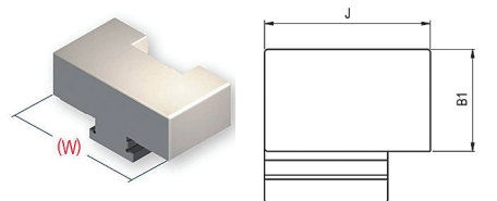
«Сырая» подвижная базовая губка art. 166 для формирования специального рабочего профиля.
