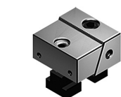
Фиксированная и подвижная гладкие губки Art.605
