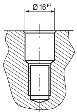
Тип Е ЗАЖИМНАЯ КОЛОННА
