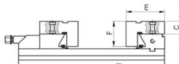
Для зажима цилиндрических заготовок. Art.131 - закаленные; Art. 131S - мягкие.
