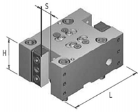
Резцедержатель для наружной обработки, двусторонний Рисунок 9
