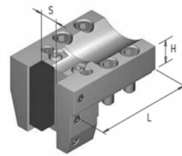
Резцедержатель для наружной обработки Рисунок 12
