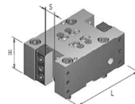
Резцедержатель для наружной обработки, двусторонний Рисунок 8
